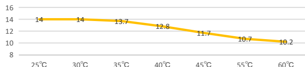
温度功率修正表 单位: kVA
